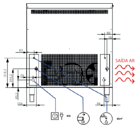
VISTA TRASEIRA
