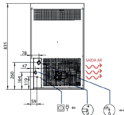
VISTA TRASEIRA
